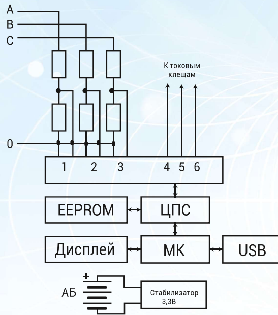
Рис. 2. Блок-схема прибора
