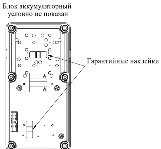
Рисунок 2 - Схема пломбировки газоанализаторов от несанкционированного доступа
