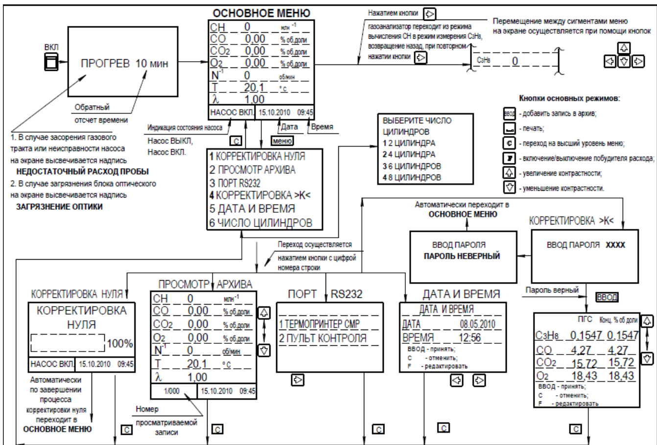
Рисунок 2.16 - Газонализатор ГИАМ-29М-1. Основное меню
