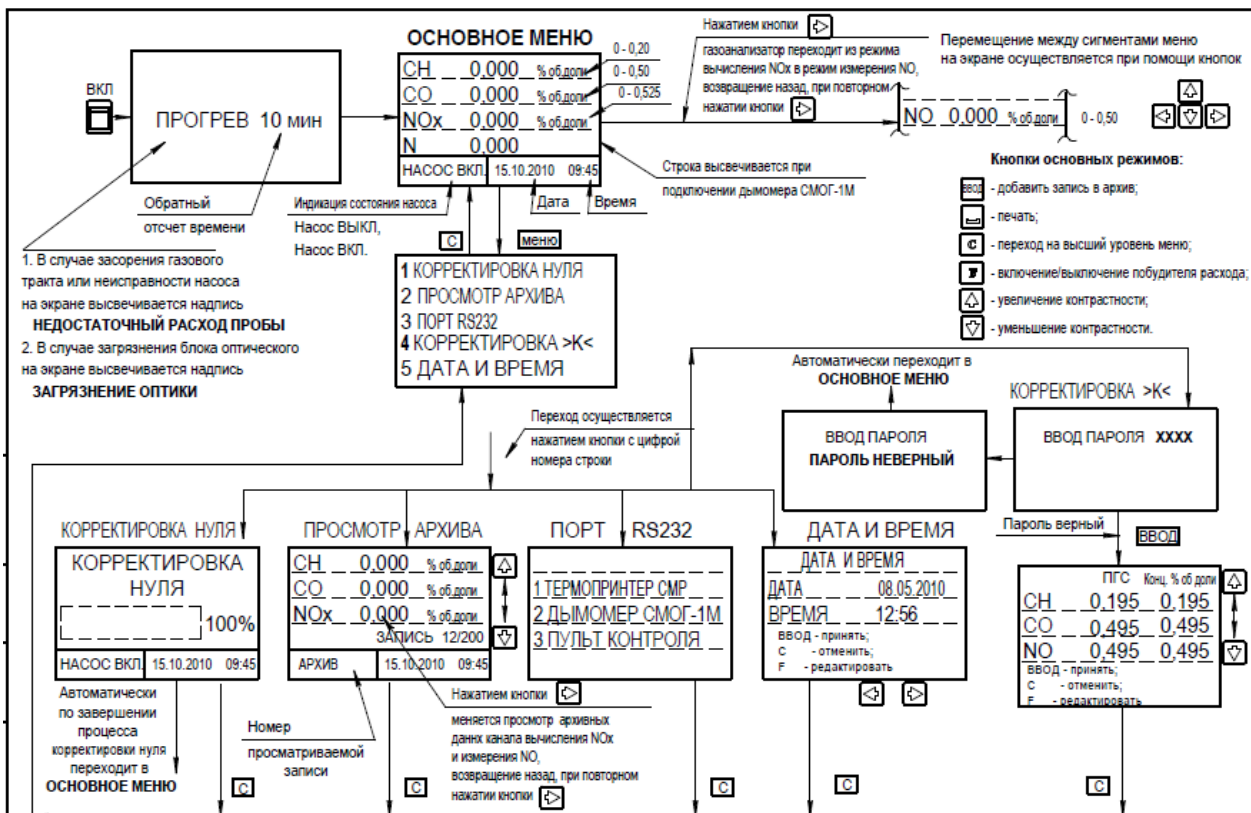
Рисунок 2.1а - Газоанализатор ГИАМ-29М-3. Основное меню
