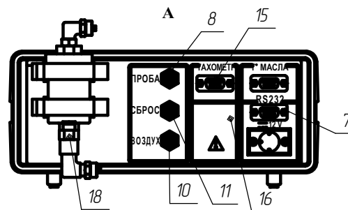
б) газоанализатор GIAM-29M-2
