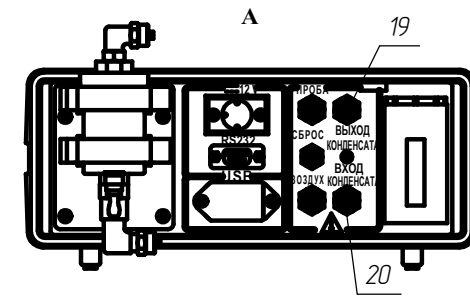
г) газоанализатор GIAM-29M-4
