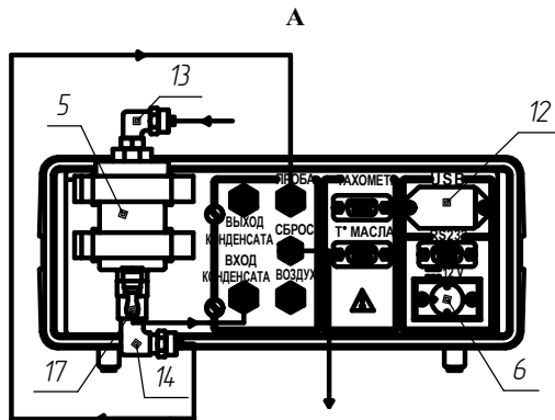
а) газоанализатор GIAM-29M-1
