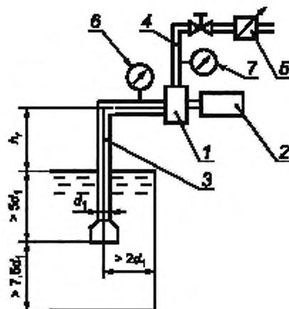
1 — насос; 2 — приводной двигатель; 3 — всасывающая линия; 4 — изпорный вентиль, 5 — устройство для измерения подачи; 6, 7 — мановакуумметры
